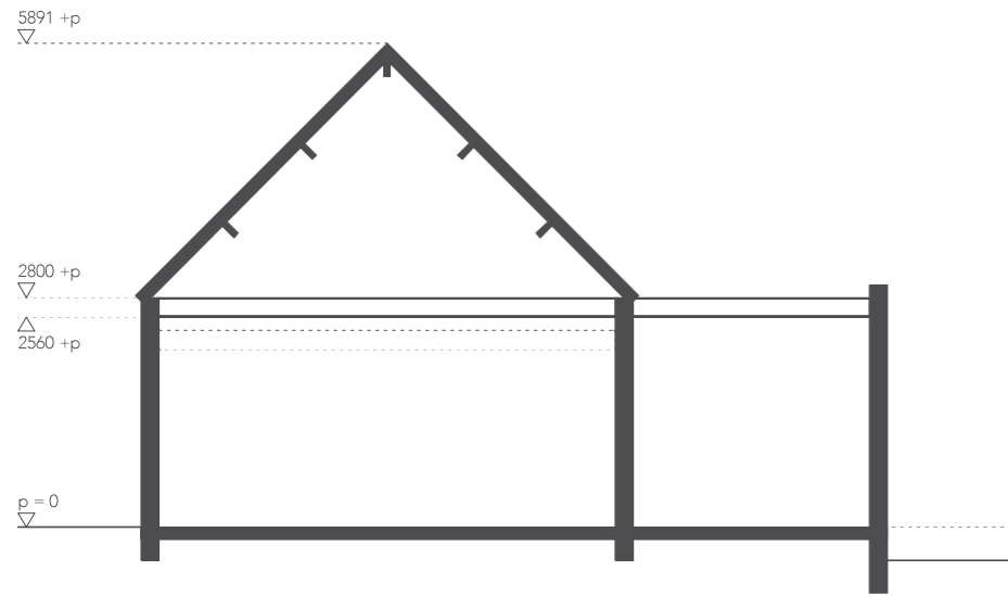
doorsnede Emmastraat 80-82
